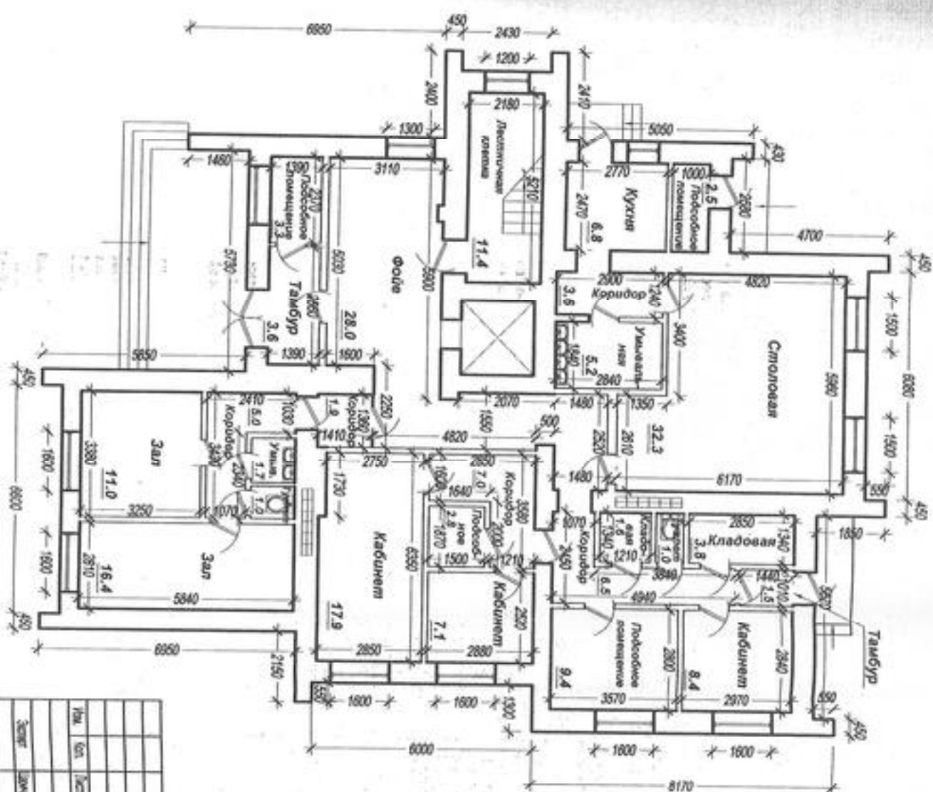
Обмерочный чертеж. План первого этажа. М 1:100.
