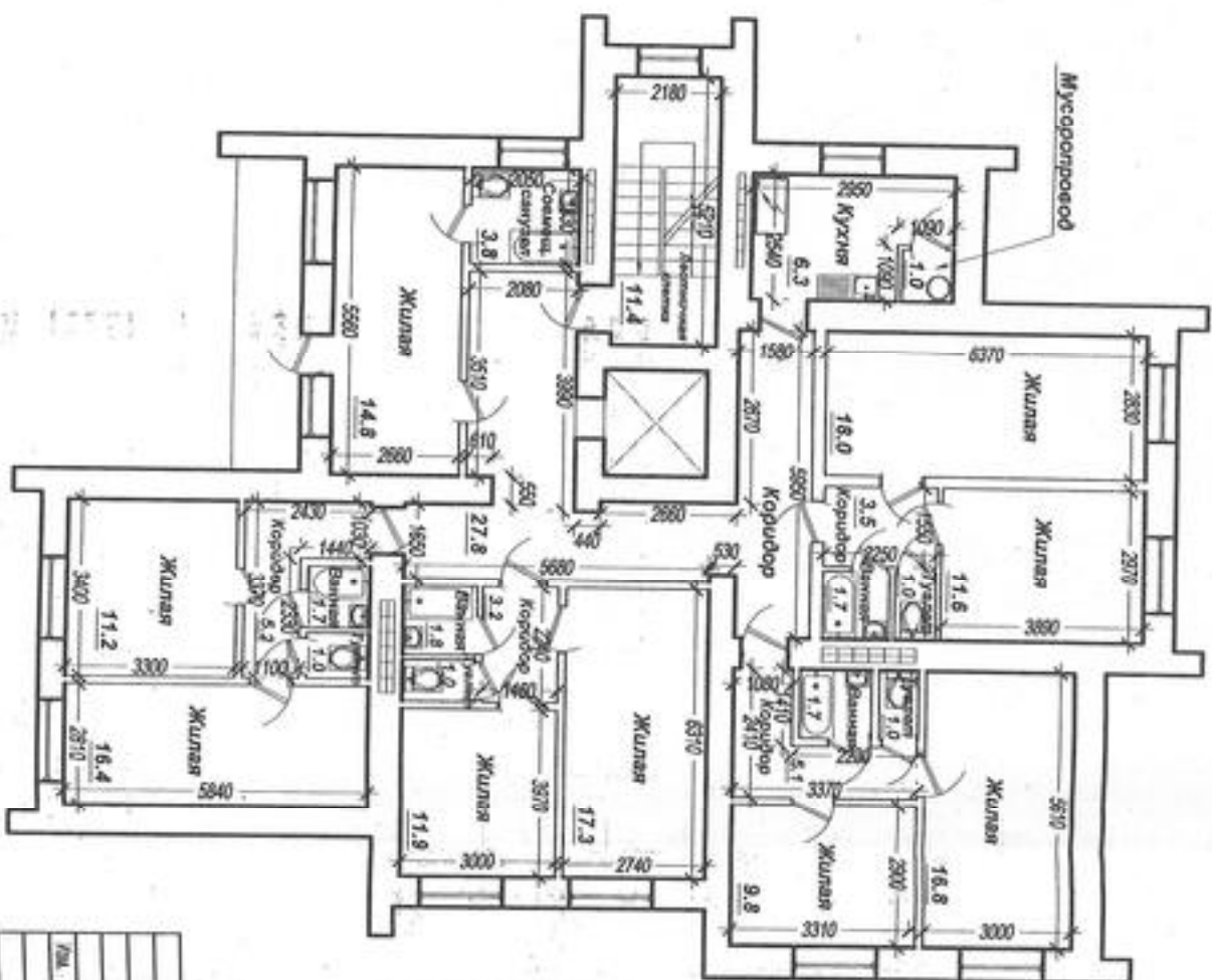
Общественный чертёж. План второго этажа. М 1:100.
